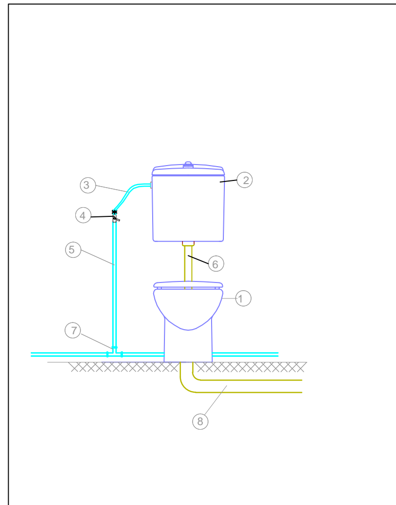
VEDERE FRONTALA
