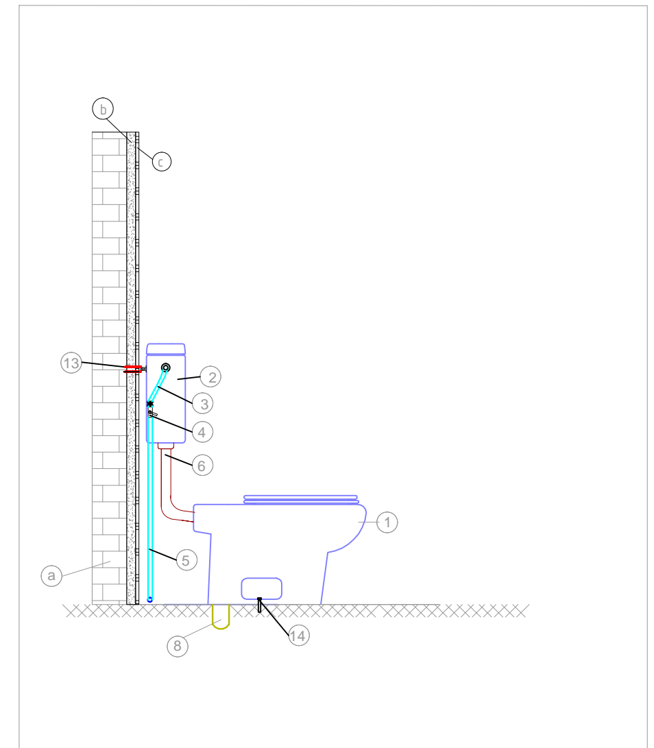
VEDERE LATERALA
